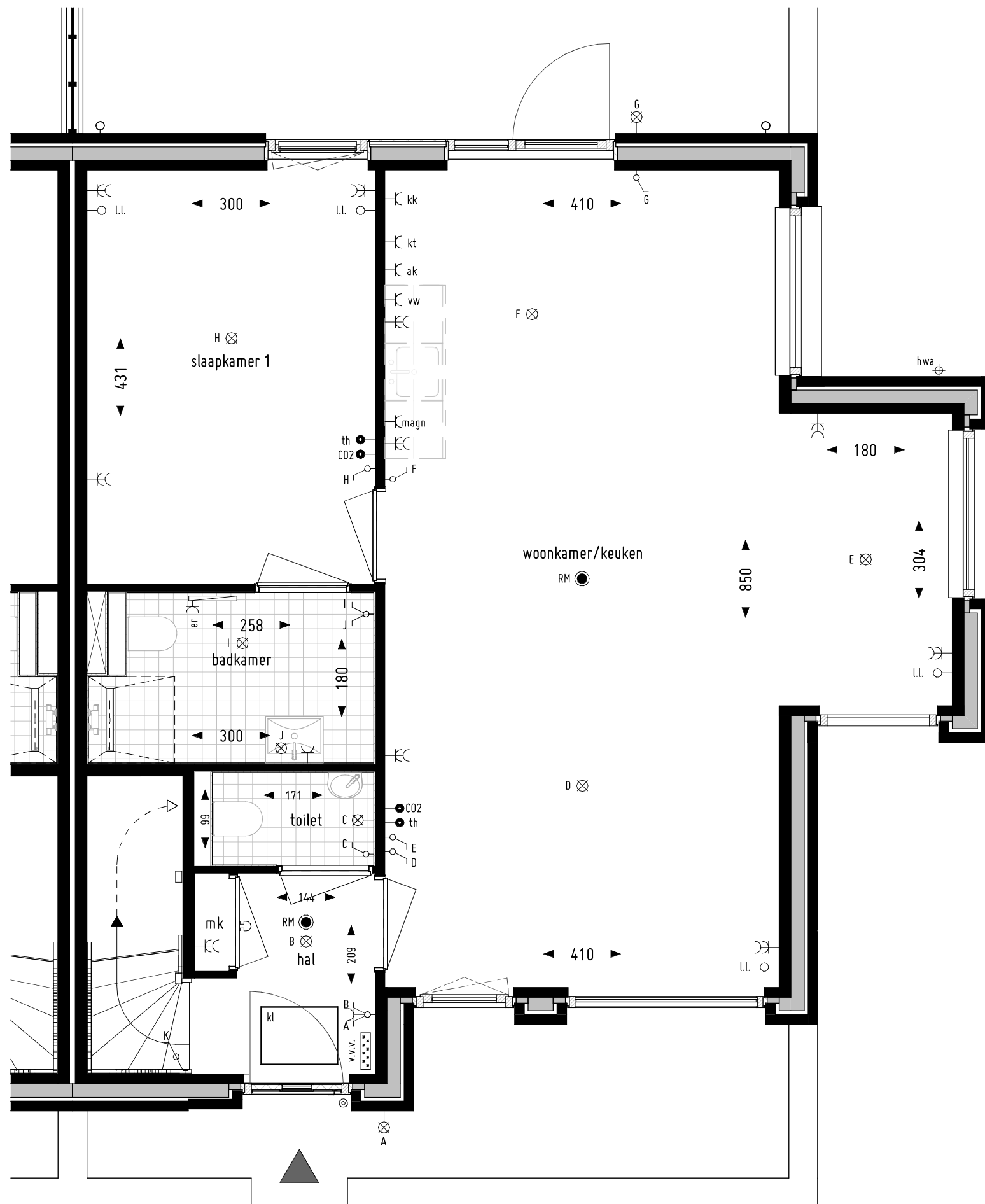
Begane grond optie erker
