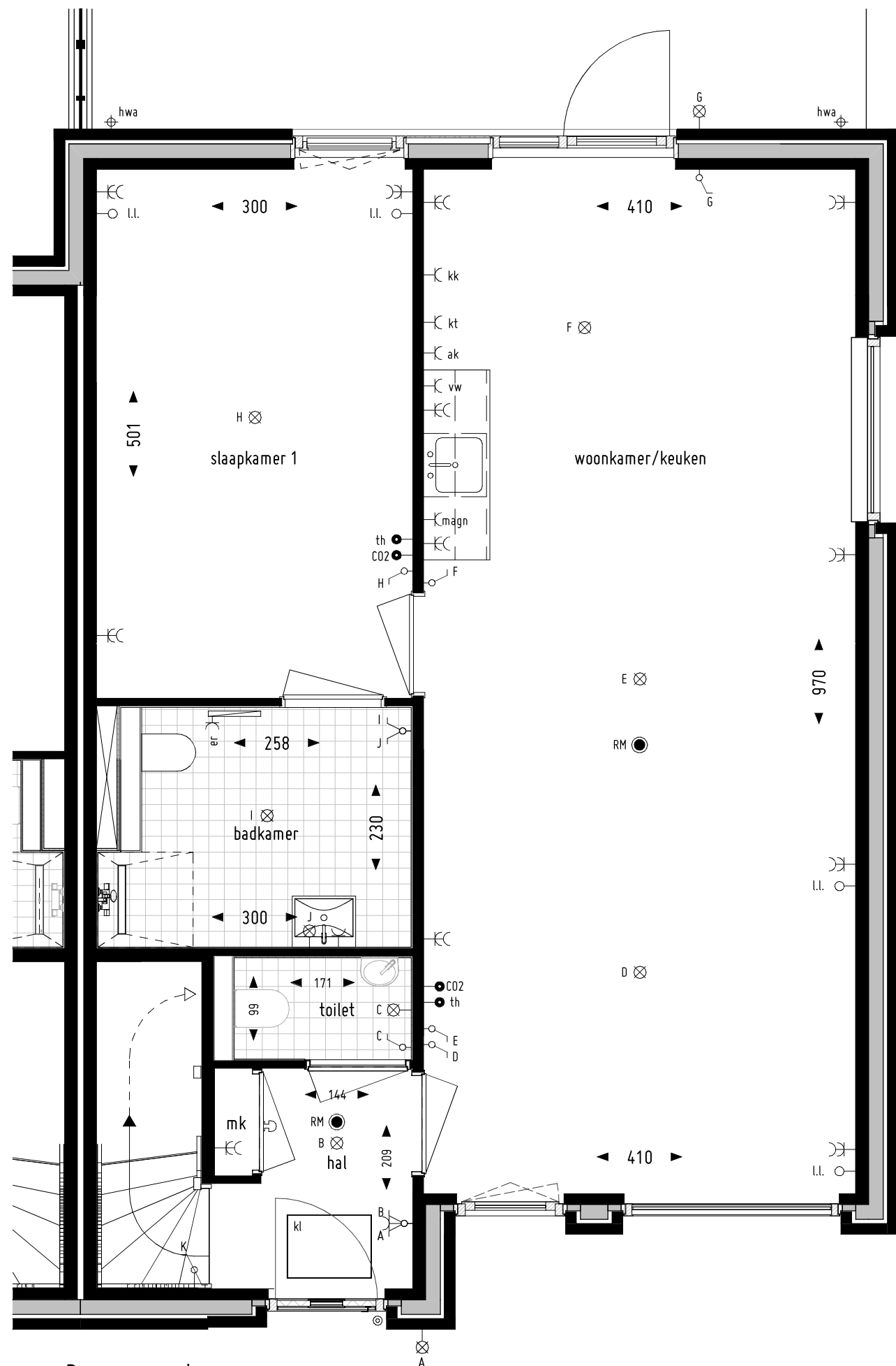
Begane grond optie uitbouw 1,2m
