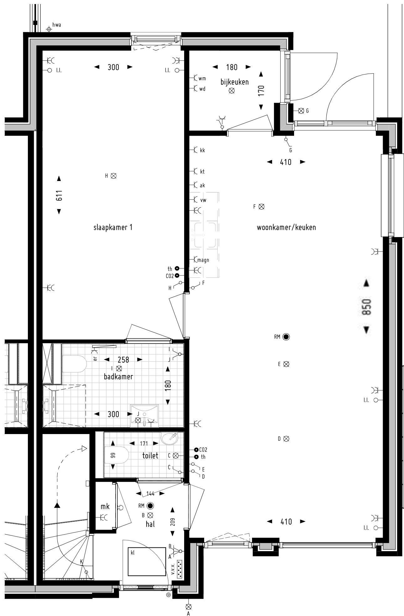
Begane grond optie bijkeuken
