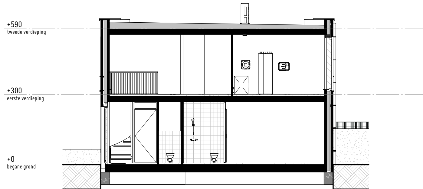
Doorsnede 1 : 100
