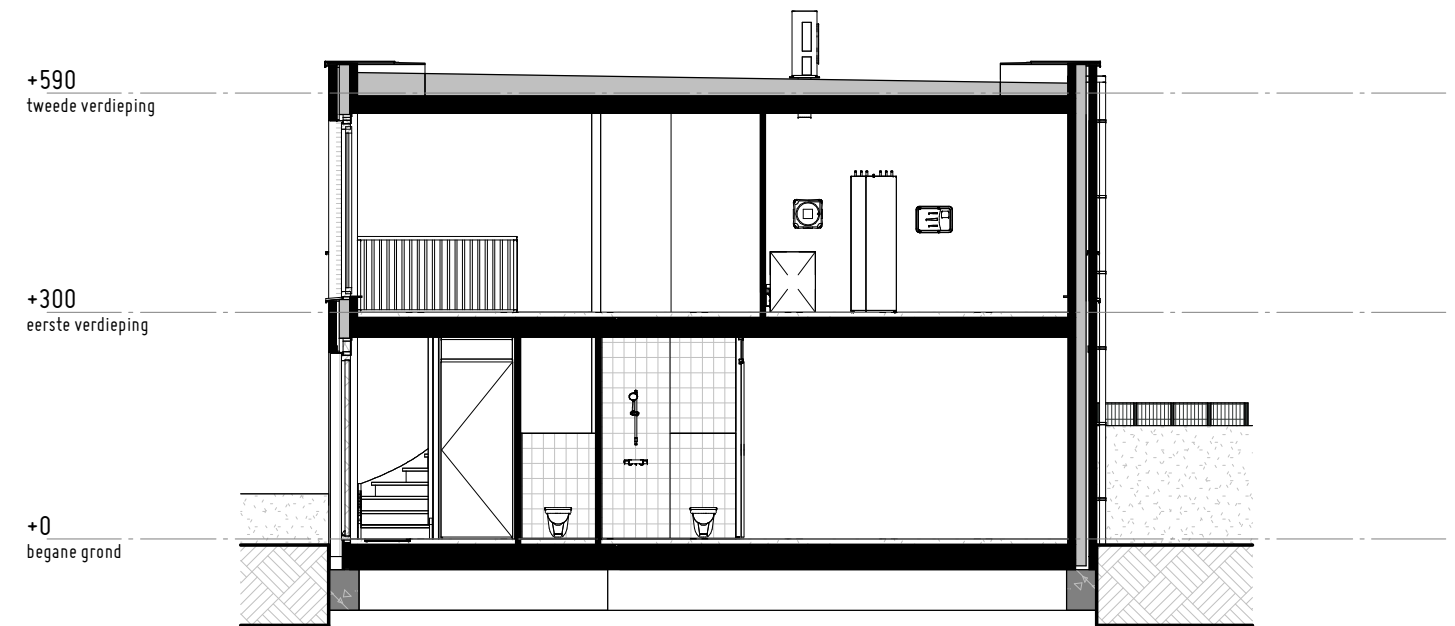
Doorsnede 1 : 100
