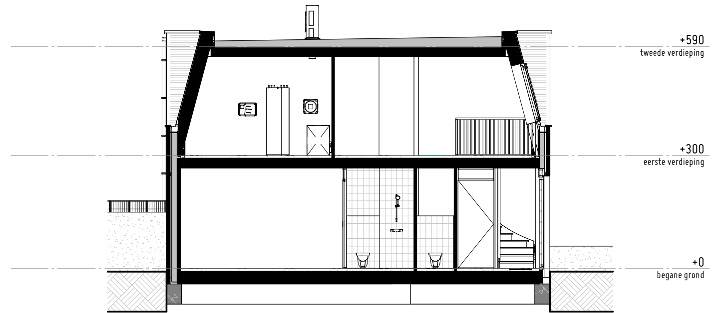
Doorsnede 1 : 100
