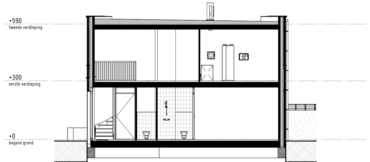
Doorsnede 1 : 100
