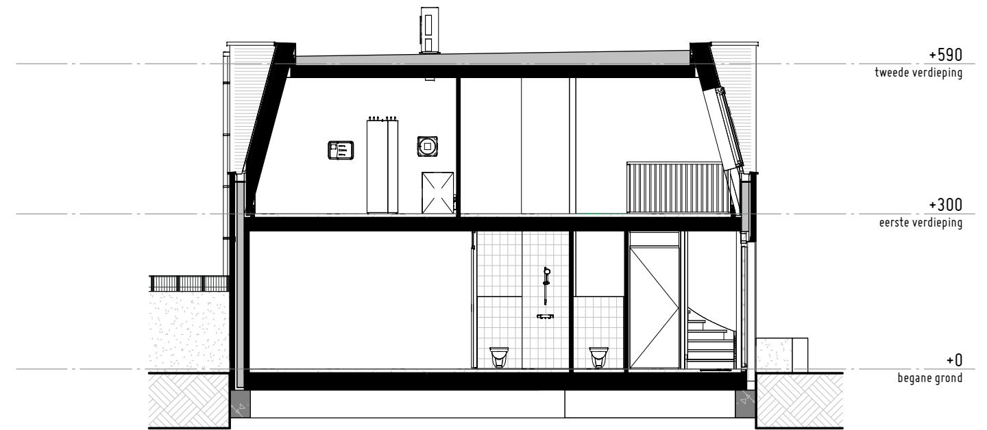
Doorsnede 1 : 100
