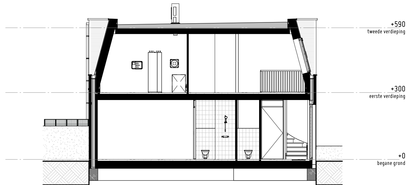
Doorsnede 1 : 100
