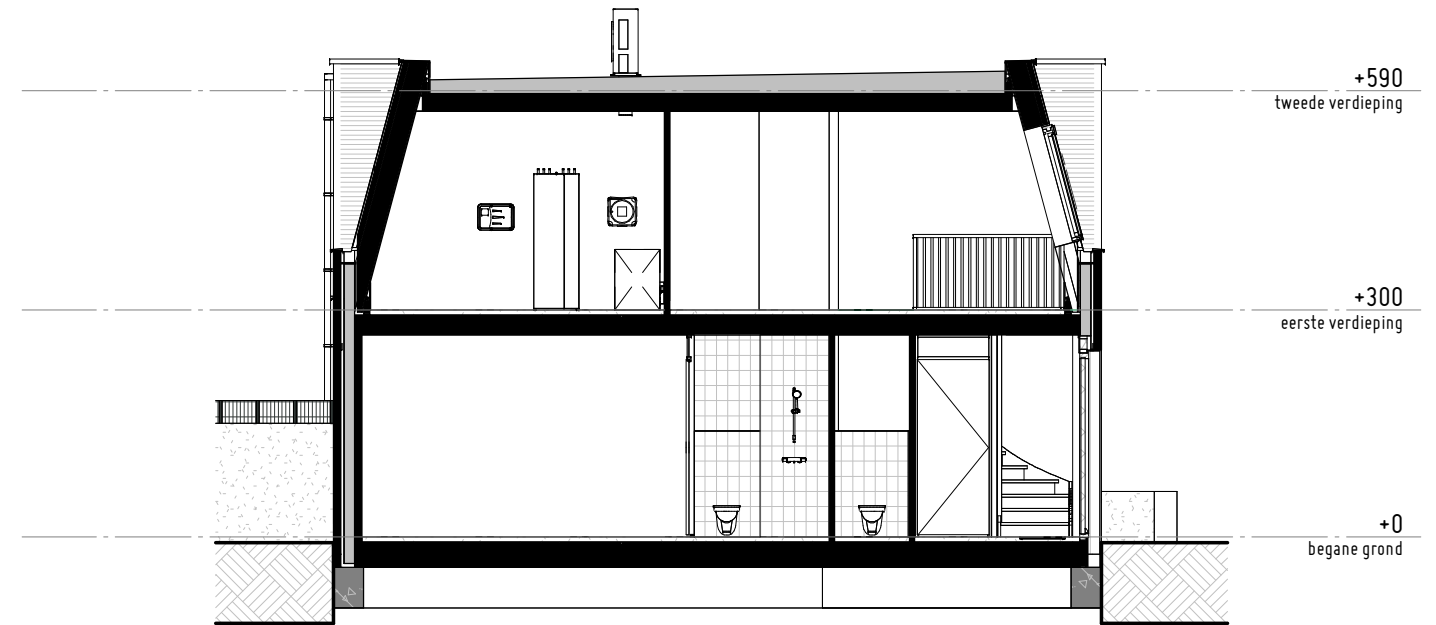
Doorsnede 1 : 100
