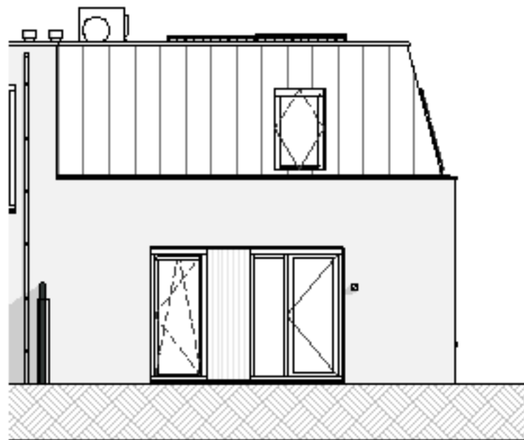
Achtergevel 1 : 100
