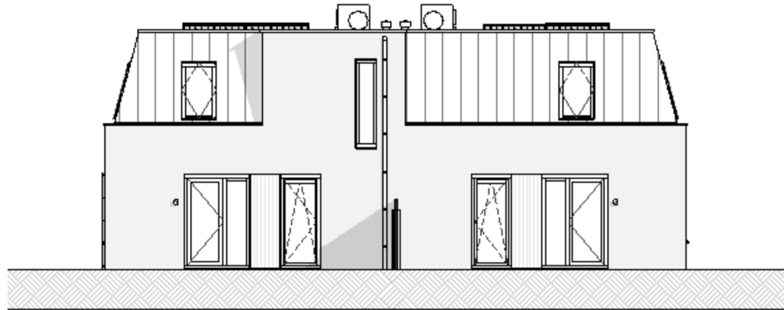
Voorgevel 1 : 100
