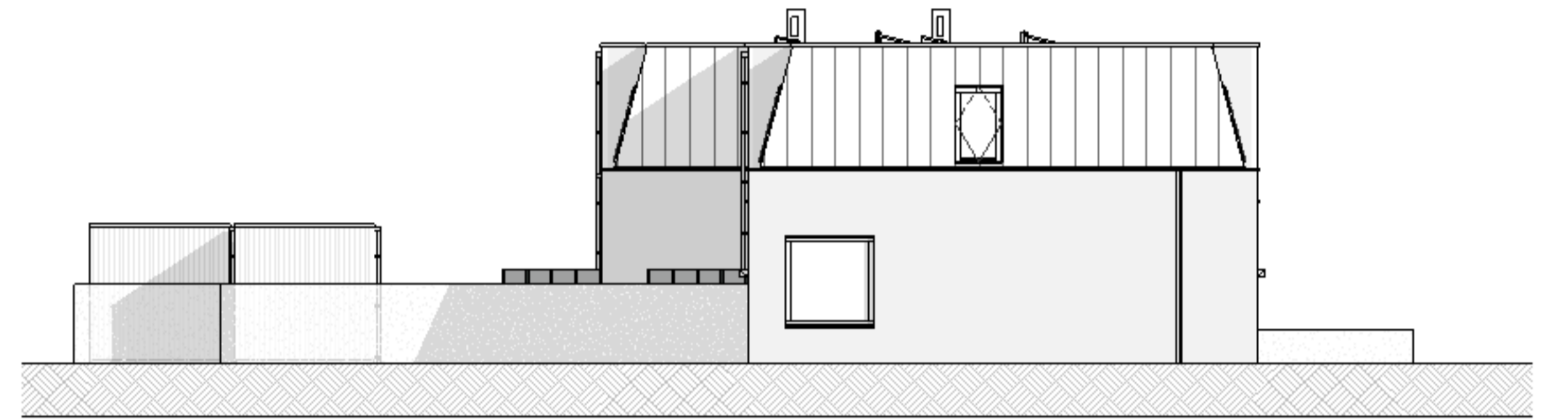
Rechter Zijgevel 1 : 100
