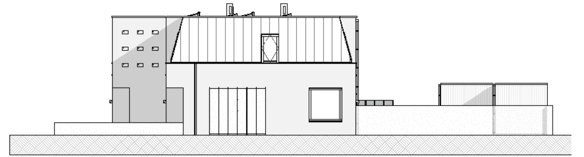
Rechter Zijgevel 1 : 100
