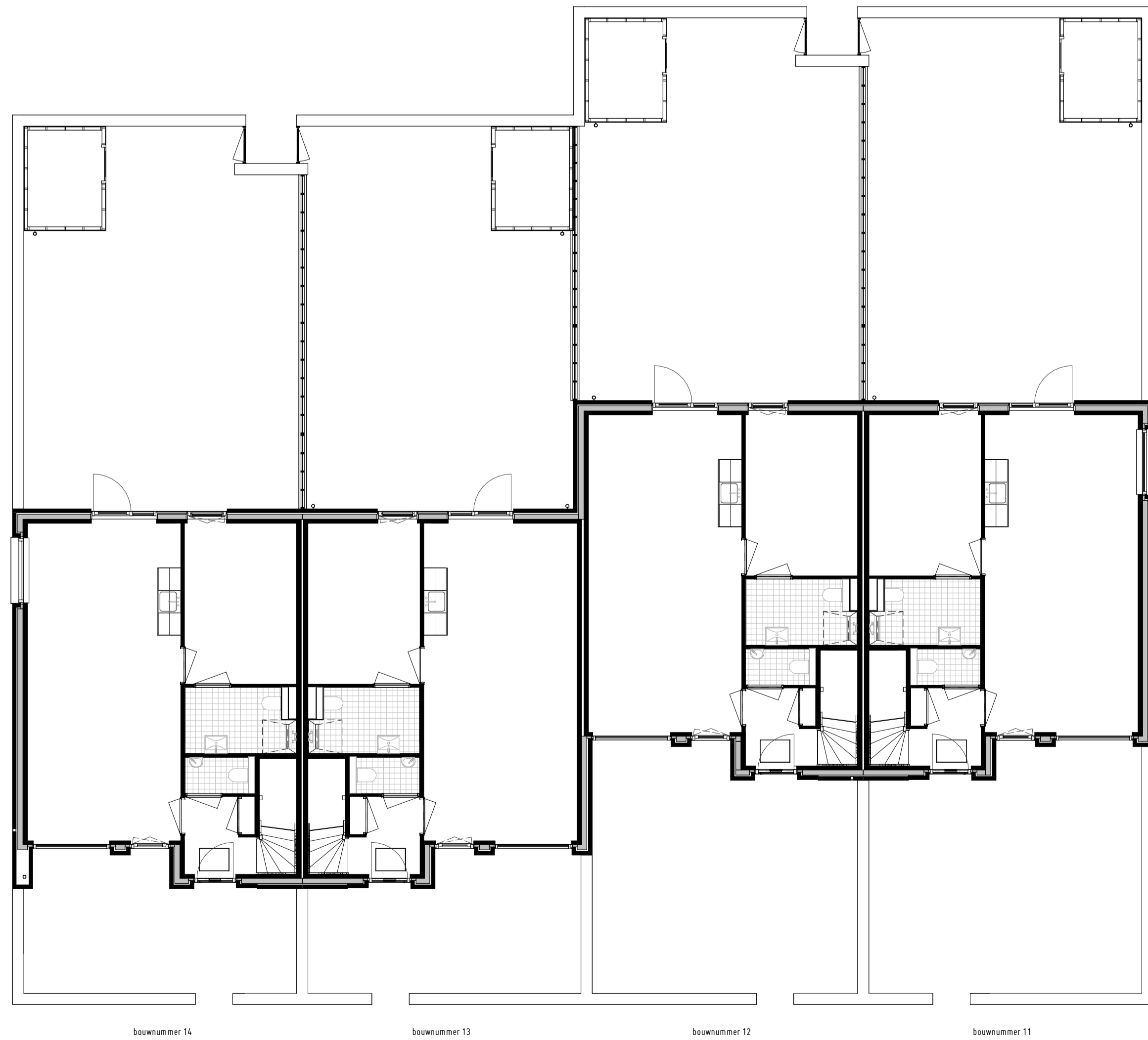
Begane grond 1 : 100
