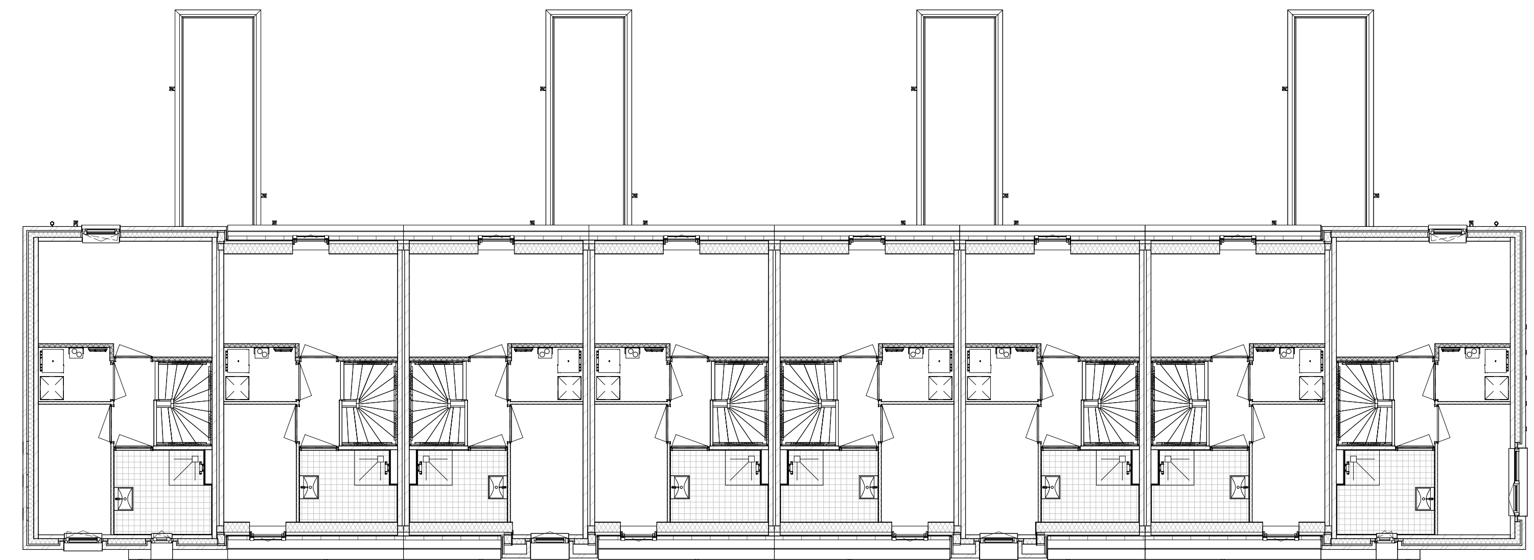
1ste verdieping 1 : 100
