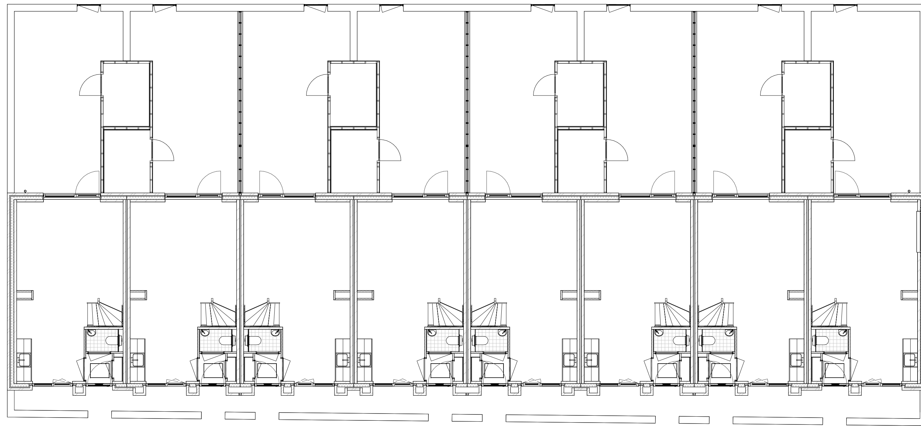
Begane grond 1 : 100
